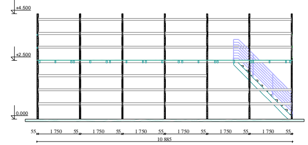
Разрез 2-2.
