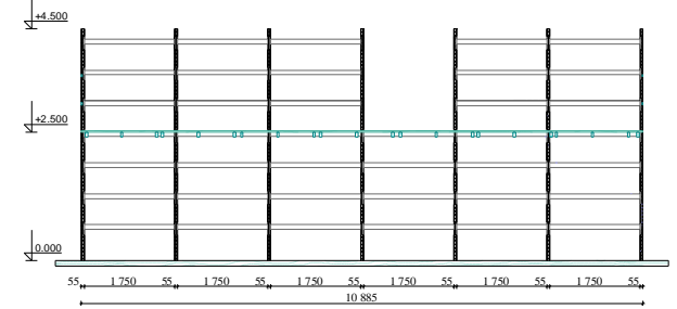
Разрез 2-2.
