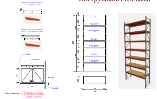
Тип грузового стеллажа.
