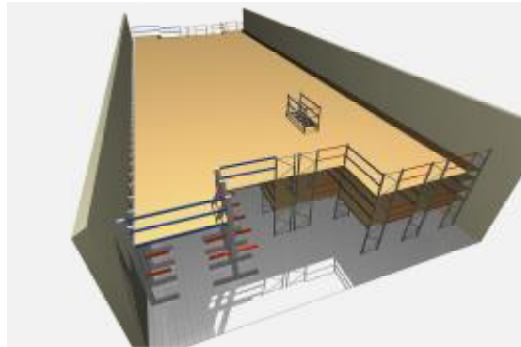
Тип грузовых и консольных стеллажей с перекрытием (Мезонин).
