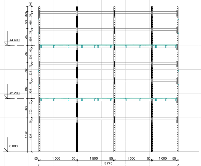
Разрез 1-1.
