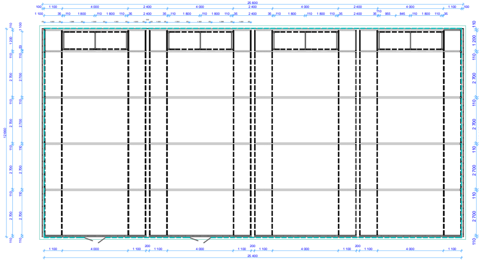
Вид 1.
