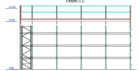
Разрез 1-1.
