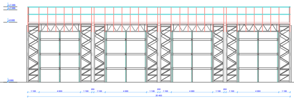
Вид 2.
