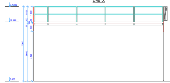
Вид 3.
