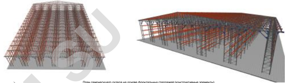
План самонесущего склада на основе фронтальных стеллажей (конструктивные элементы).
